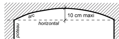
Fig. D Hauteur des linteaux cintrés
