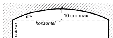
Fig. Z Hauteur des linteaux cintrés
