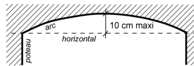
Fig. L Hauteur des linteaux cintrés
